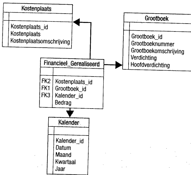
Afbeelding 11: Datamodel.
