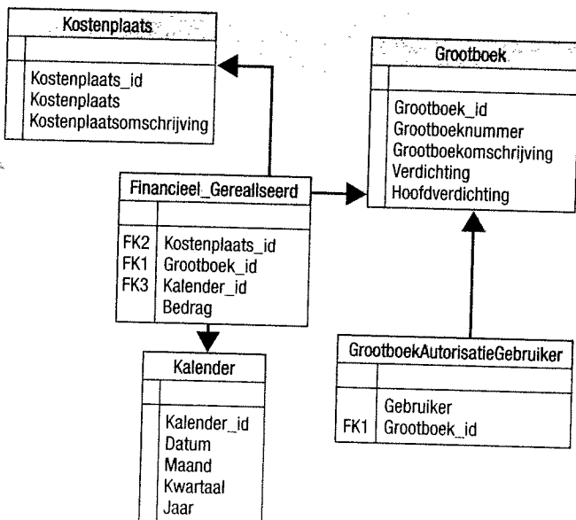
Afbeelding 12: Aangepast datamodel.
